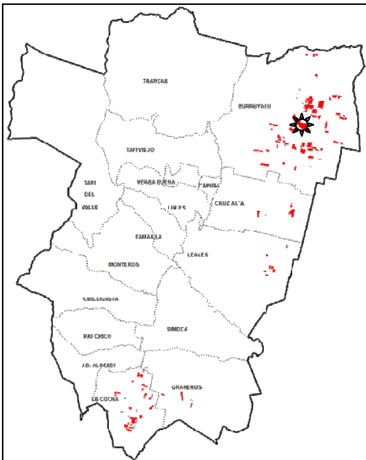
Figura 2. Mapa del área garbancera de Tucumán y sitio donde se realiza el relevamiento de la oruga bolillera ( Helicoverpa spp.) en el cultivo de garbanzo. Fuente: Sección Sensores Remotos y SIG (EEAOC).
