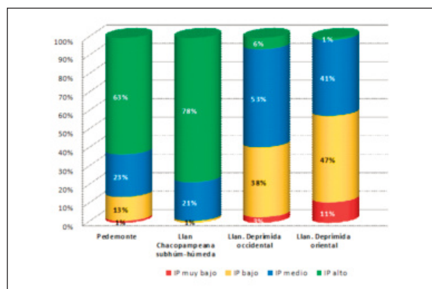
Figura 1. Distribución porcentual de Índices de Productividad de 2550 suelos en las distintas regiones cañeras de la provincia de Tucumán- Argentina
